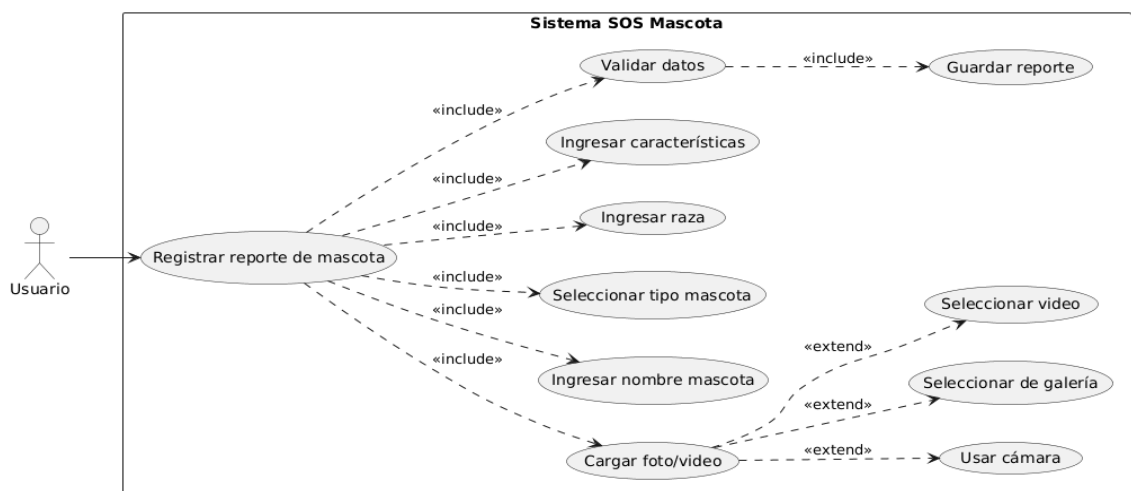
Figura 04. Diagrama de Caso de Uso 004: Registrar reporte de mascota
